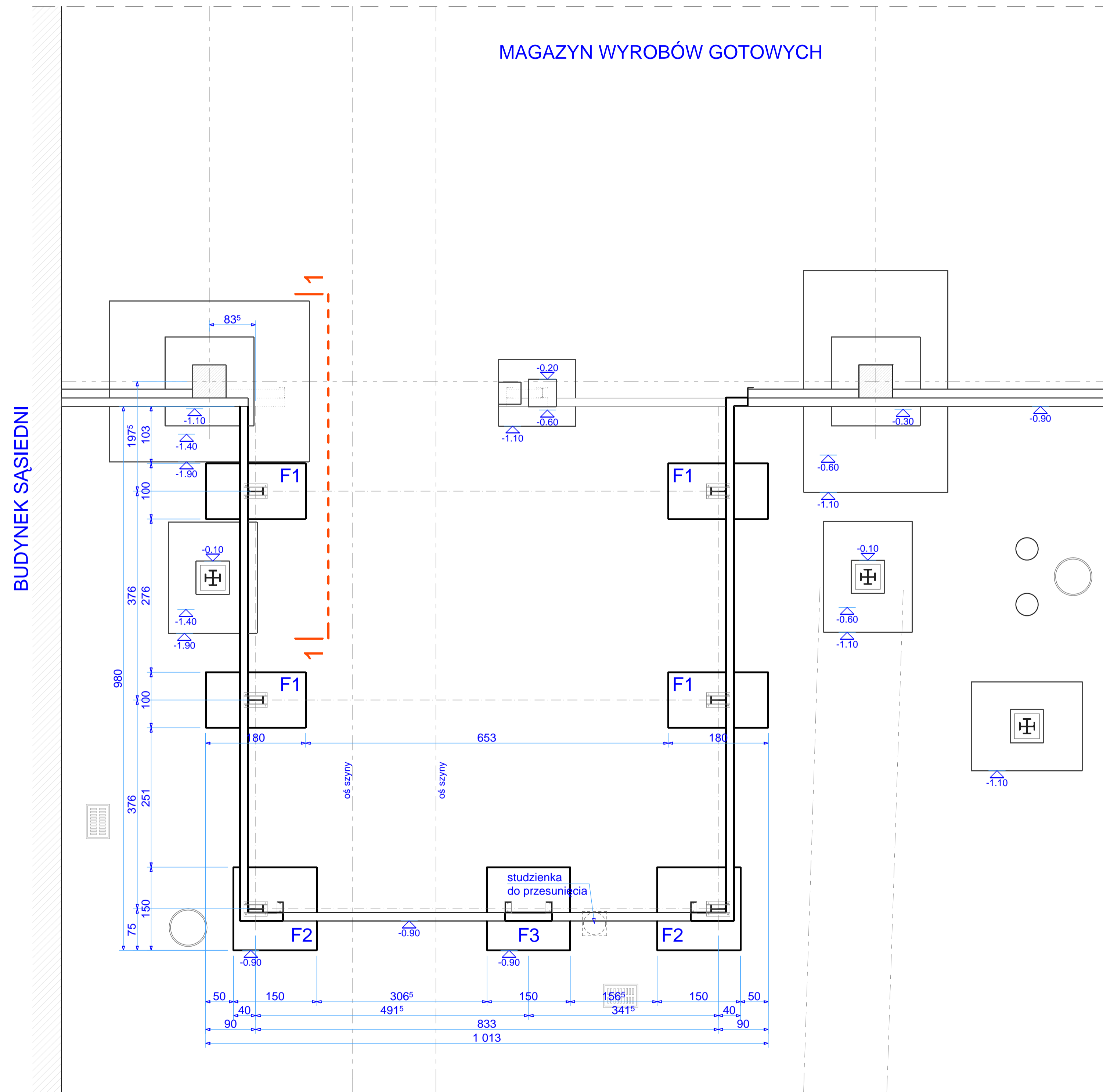
RZUT FUNDAMENTÓW 1:50
